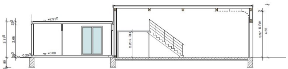
Schnitt 1-1
